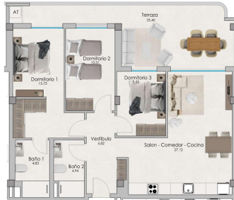
PLANTA PISO 1 / ESCALERA 1 VIVIENDA 4
