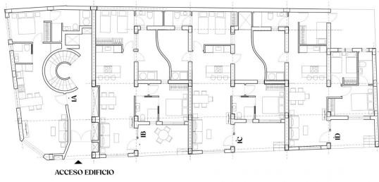
PLANTA I
